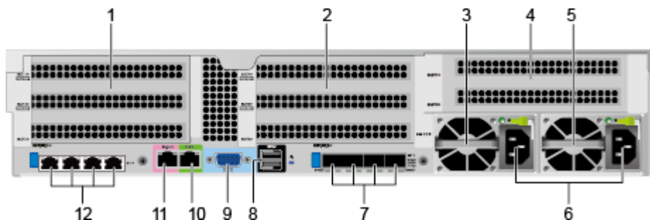
图 2-10 后面板组件
