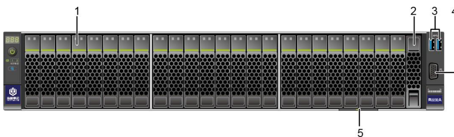
图 2-4 24x2.5 SAS/SATA 直通硬盘配置前面板组件
