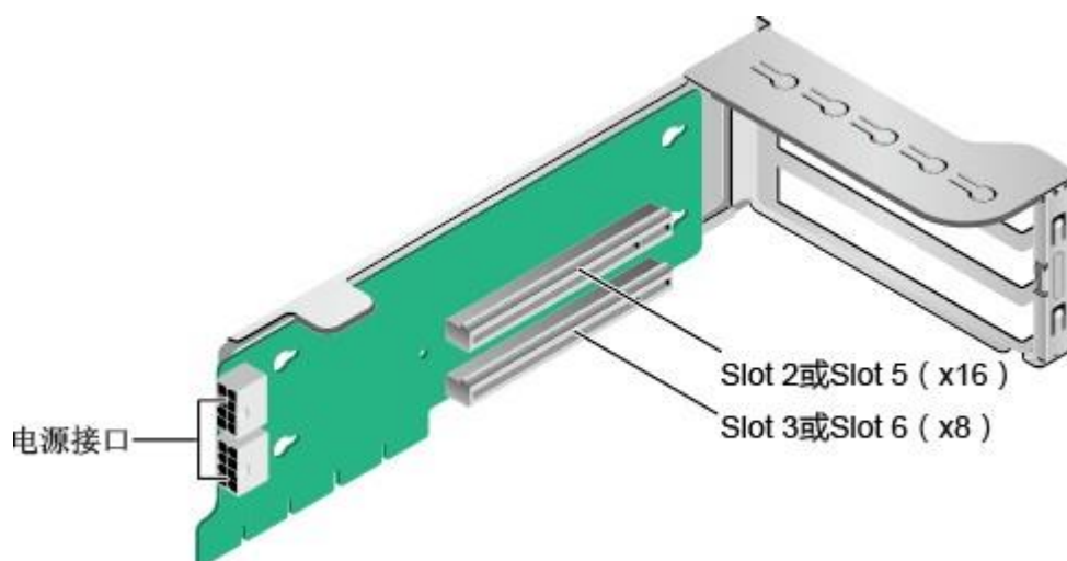
图 2-22 Riser 卡 2 (1x8+1x16)
