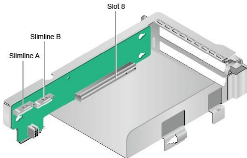
图 2-27 Riser 卡 7 (1x16)
