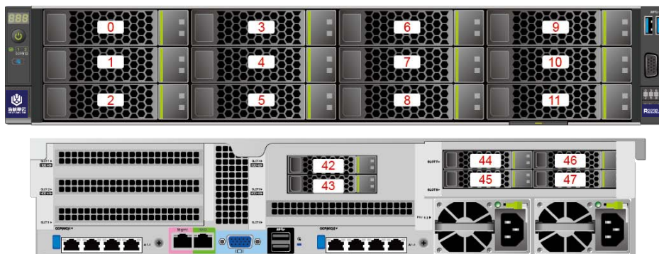
图 2-15 12x3.5 英寸硬盘直通配置
