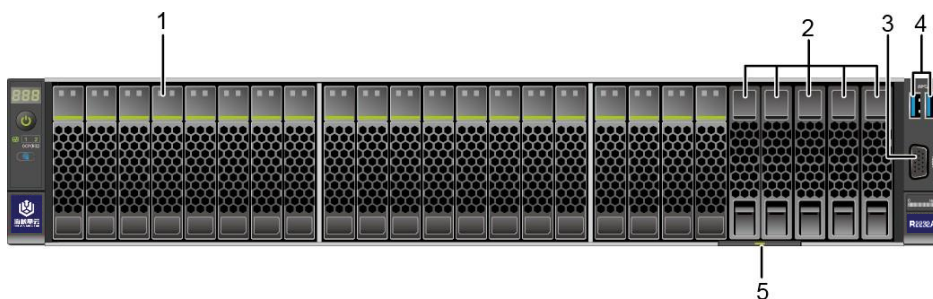
图 2-3 8x2.5 SAS/SATA+12x2.5 NVMe 硬盘配置前面板组件
