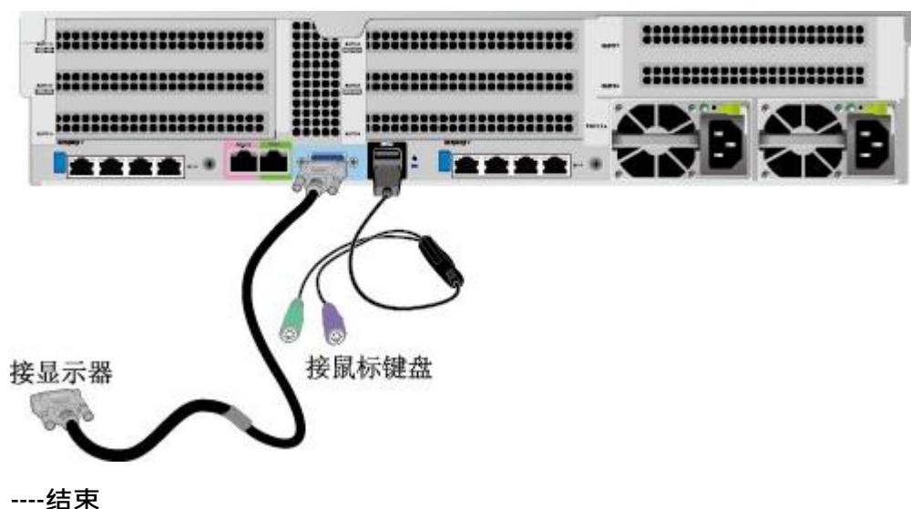
图 5-16 连接 USB 转 PS2 线缆和 VGA 接口
