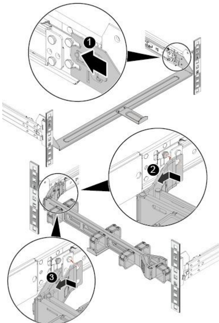
图 5-15 安装理线架
