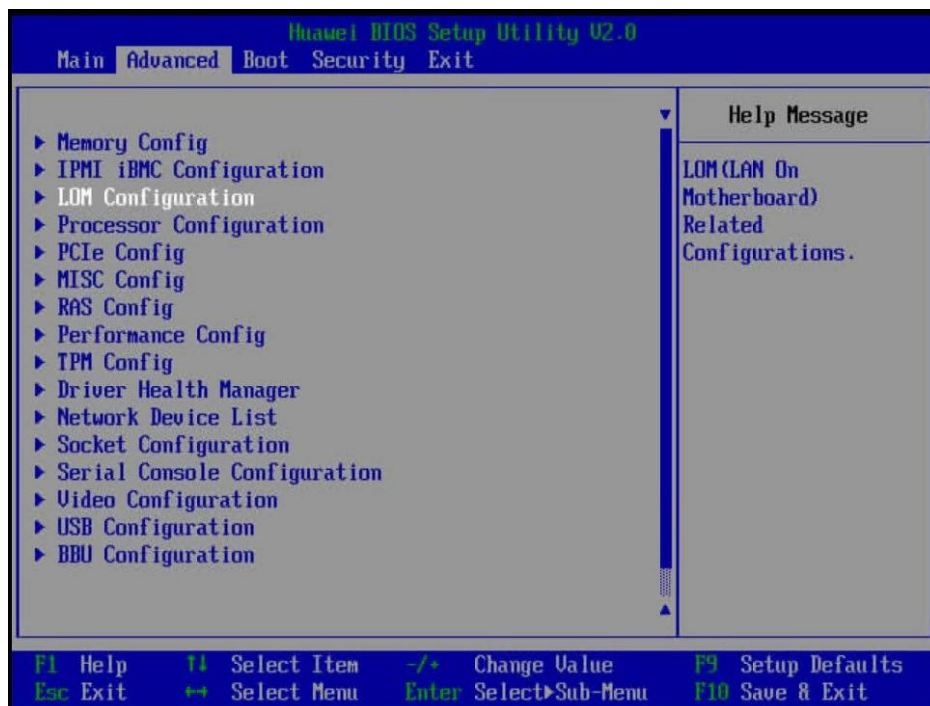
图 5-48 “Advanced” 界面
