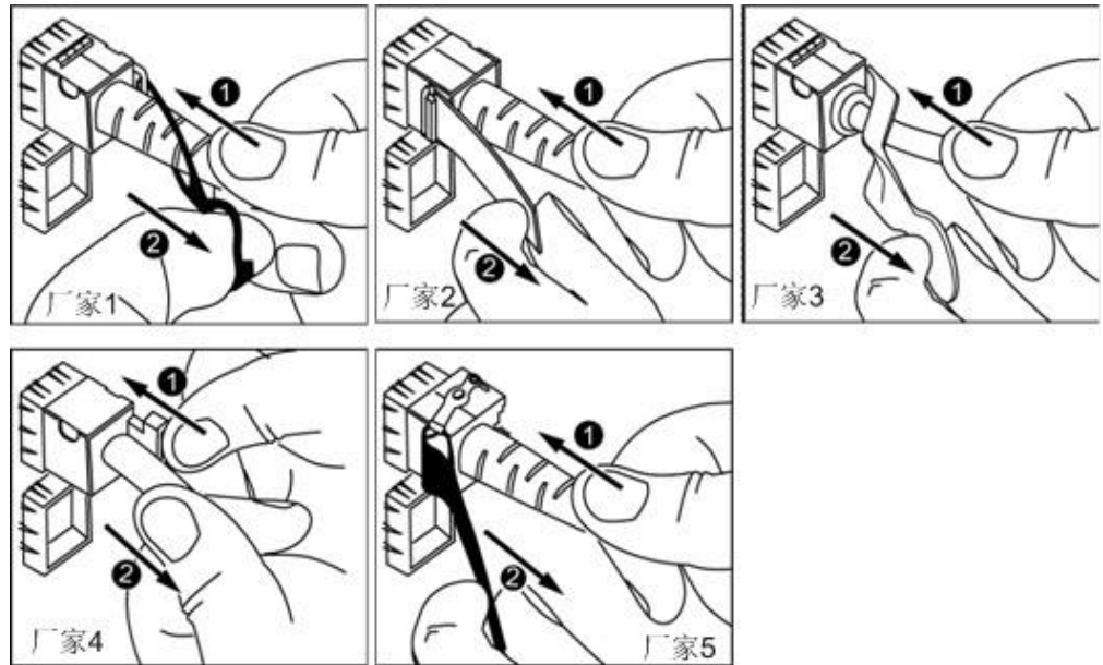
图 5-19 拔出 SFP+电缆
