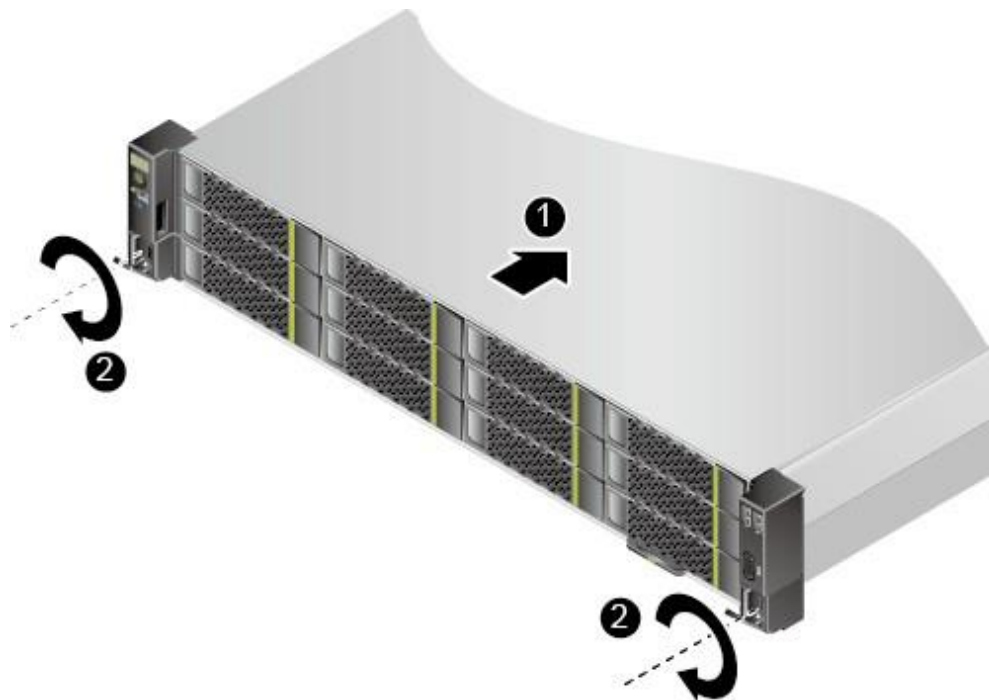
图 5-9 安装服务器
