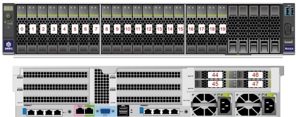
图 2-17 8x2.5 SAS/SATA+12x2.5 NVMe 硬盘配置硬盘编号
