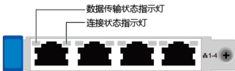
图 2-12 TM210 (4xGE 电口)
