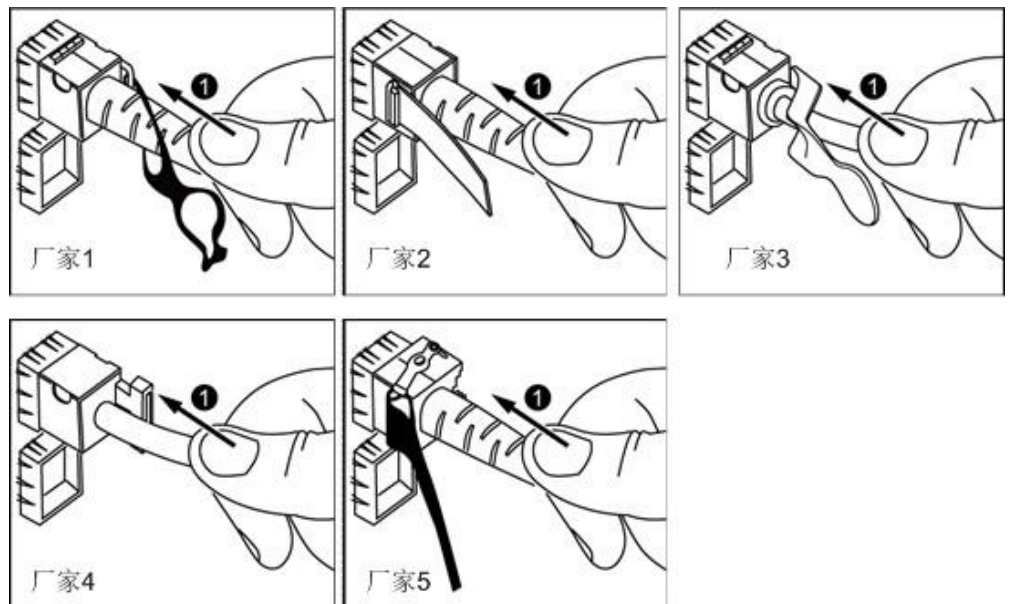
图 5-20 连接 SFP+电缆
