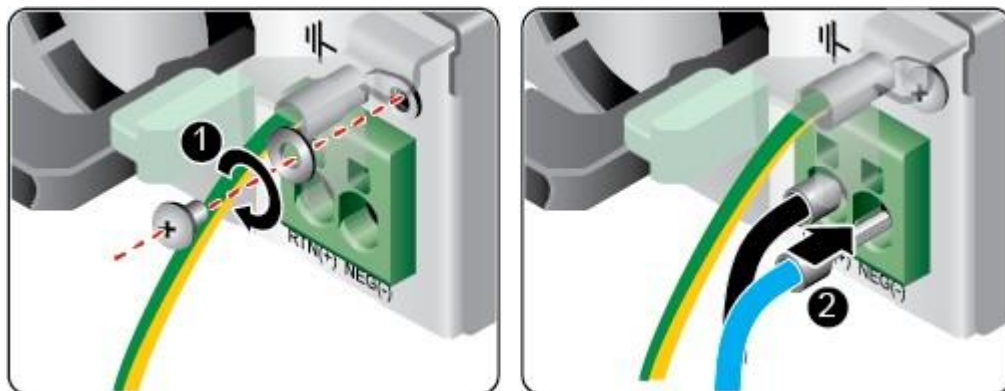
图 5-25 连接线缆
