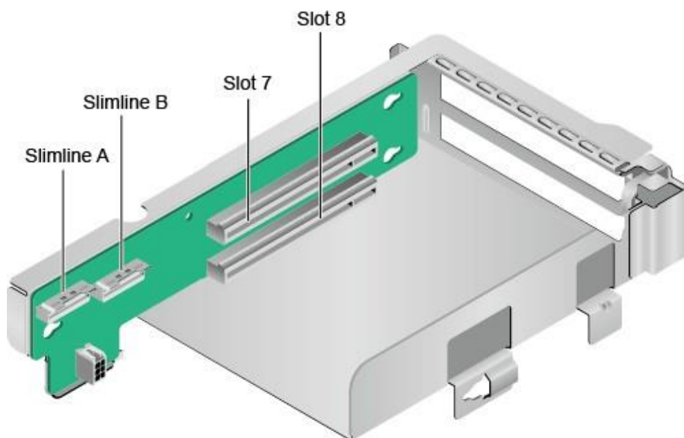
图 2-26 Riser 卡 6 (2x8)
