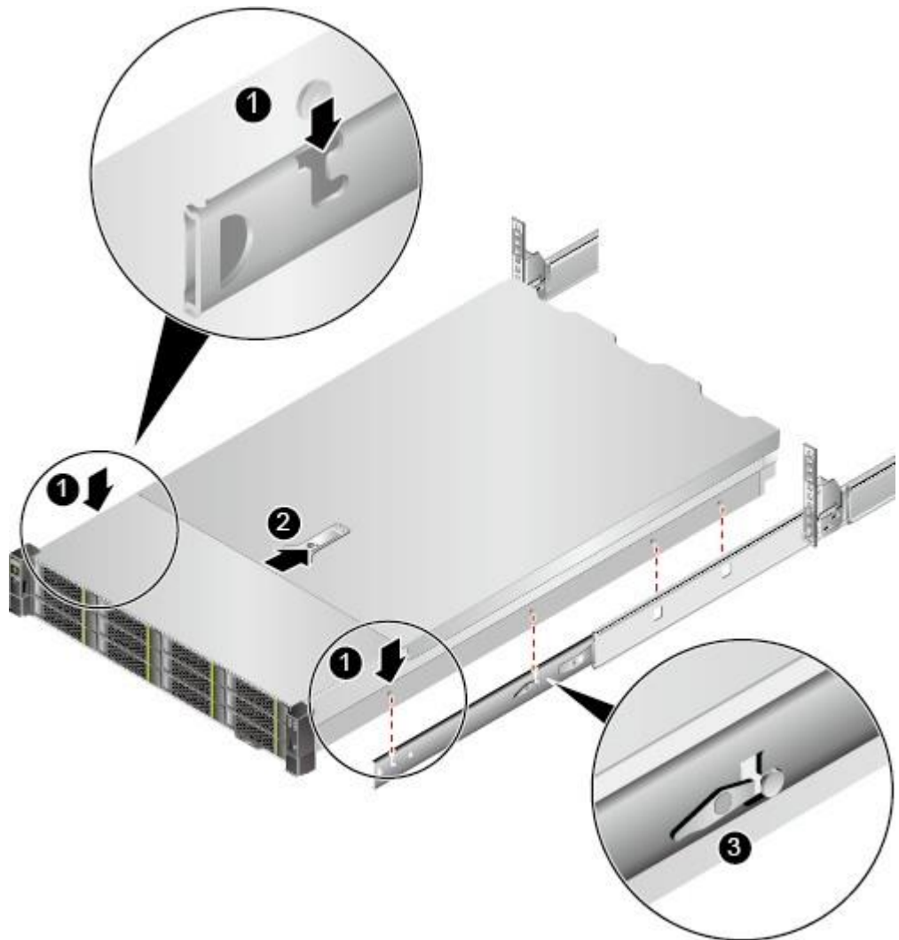
图 5-12 安装服务器
