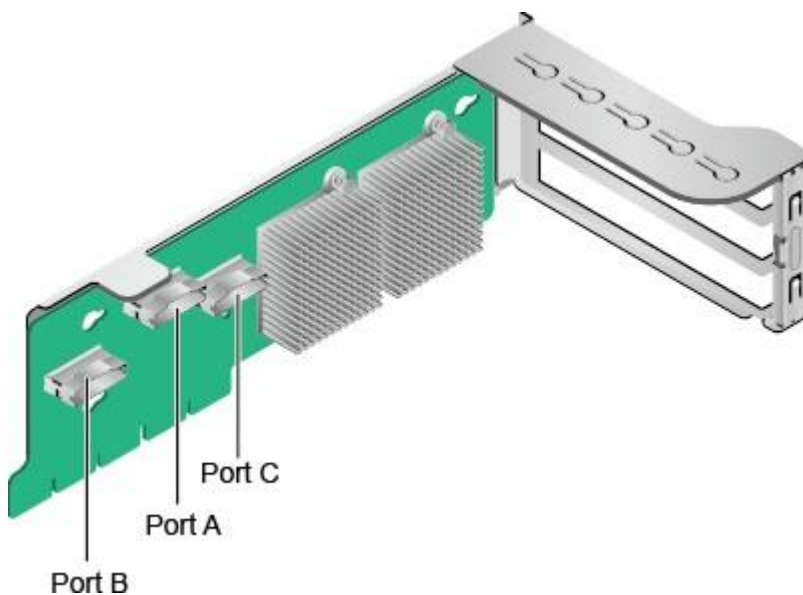
图 2-23 Riser 卡 3 (12NVMe 专用)
