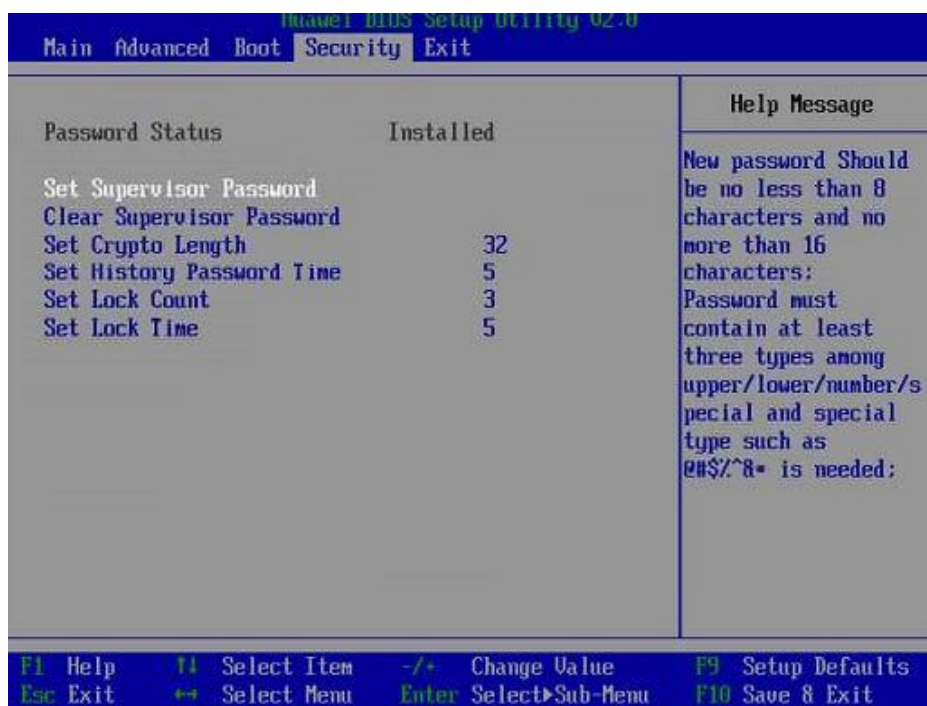
图 5-50 “Security”界面
