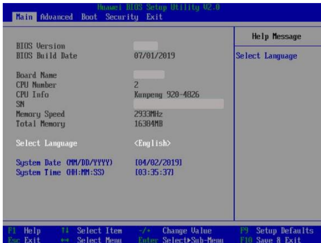
图 5-51 “Main”界面
