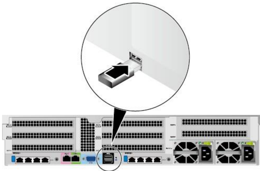
图 5-21 连接 USB 接口
