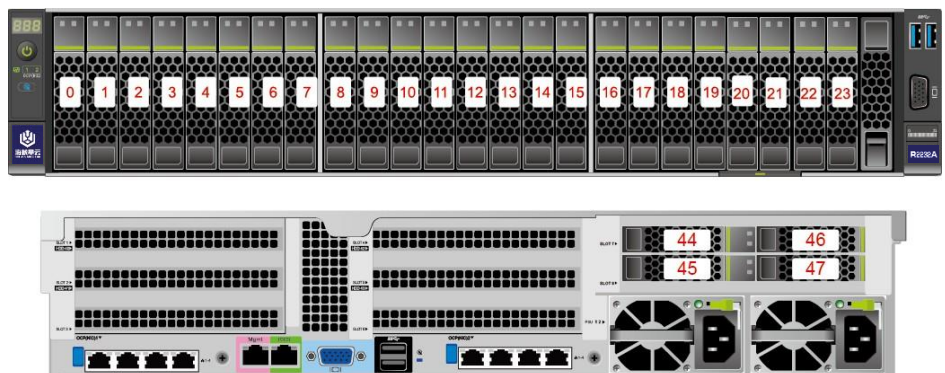
图 2-18 24x2.5 SAS/SATA 直通硬盘配置
