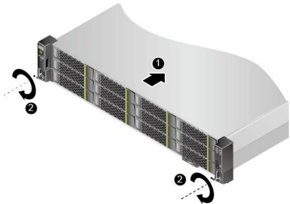
图 5-7 安装服务器
