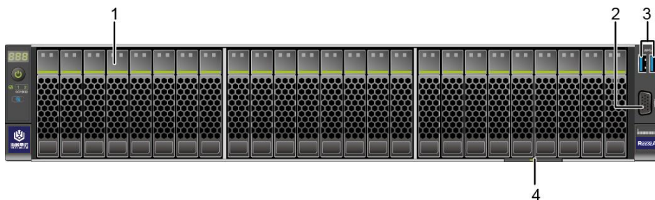
图 2-2 25x2.5 英寸硬盘配置前面板组件
