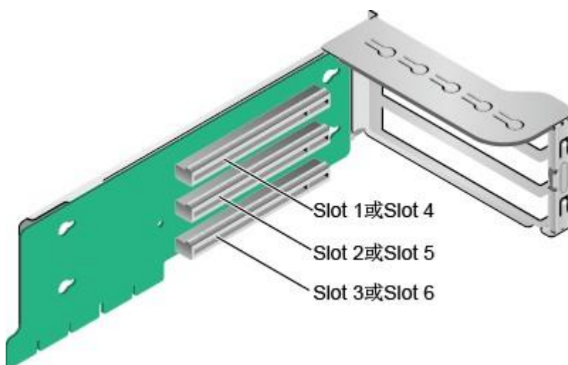
图 2-21 Riser 卡 1 (3x8)
