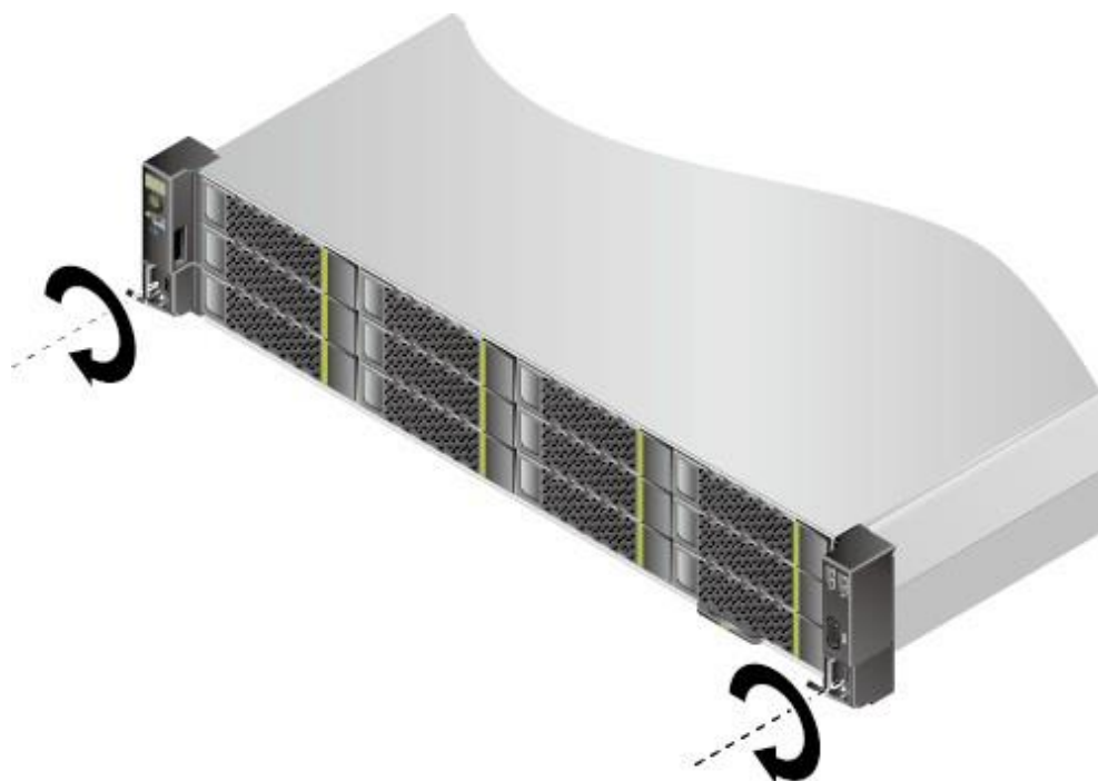
5-14 固定服务器
