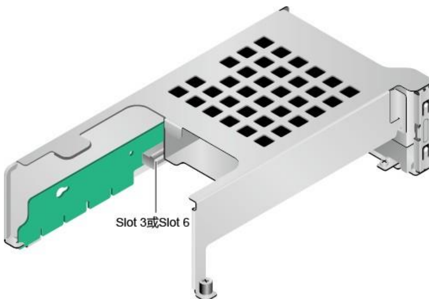
图 2-24 Riser 卡 4 (1x16)
