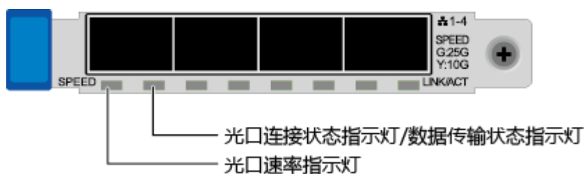
图 2-13 TM280 (4x25GE 光口)
